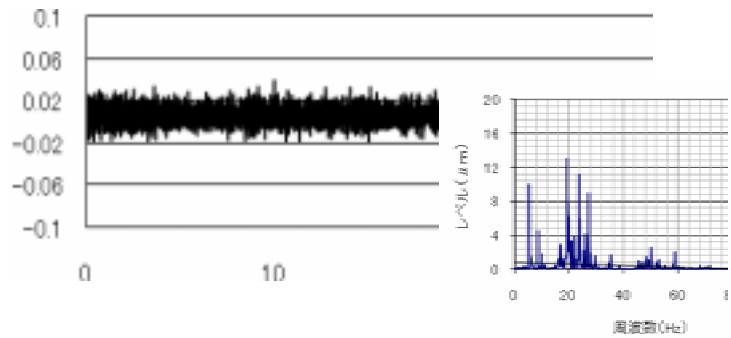
振動波形と周波数分析
